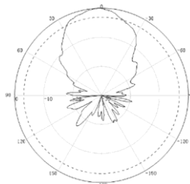
Vertical 2700MHz
