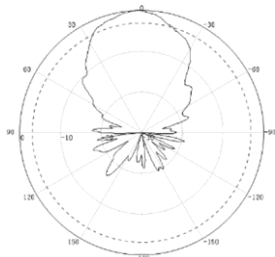
Vertical 2700MHz
